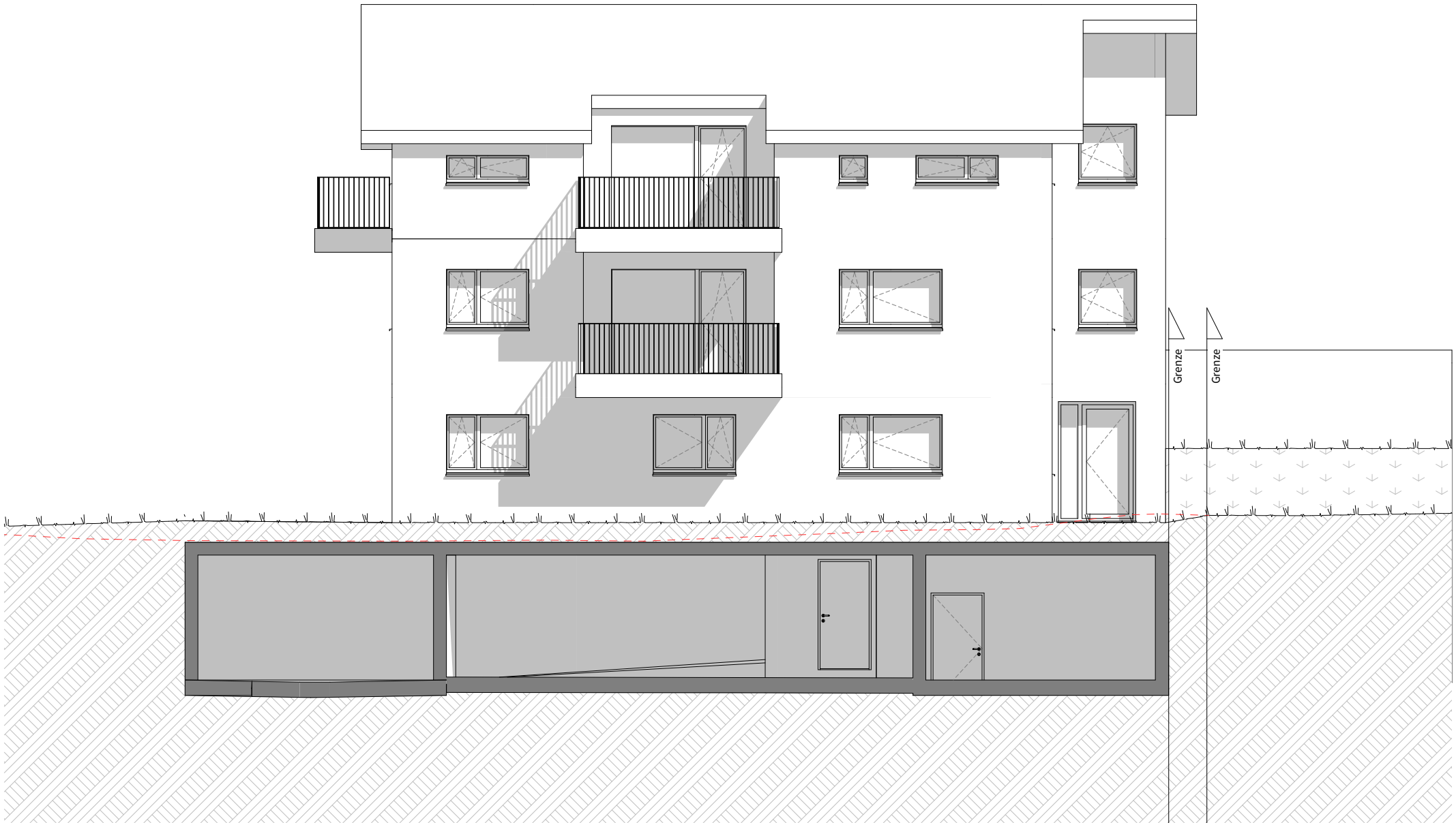
Ostansicht
